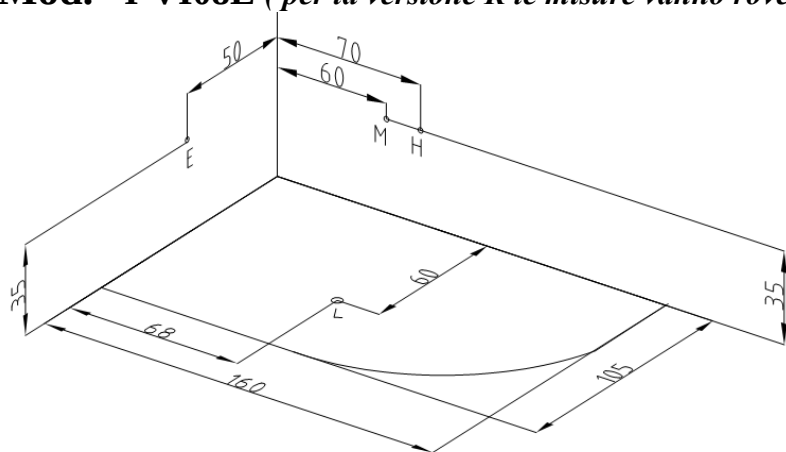
Mod. I-VI08L ( per la versione R le misure vanno rovesciate dall'altro lato )
